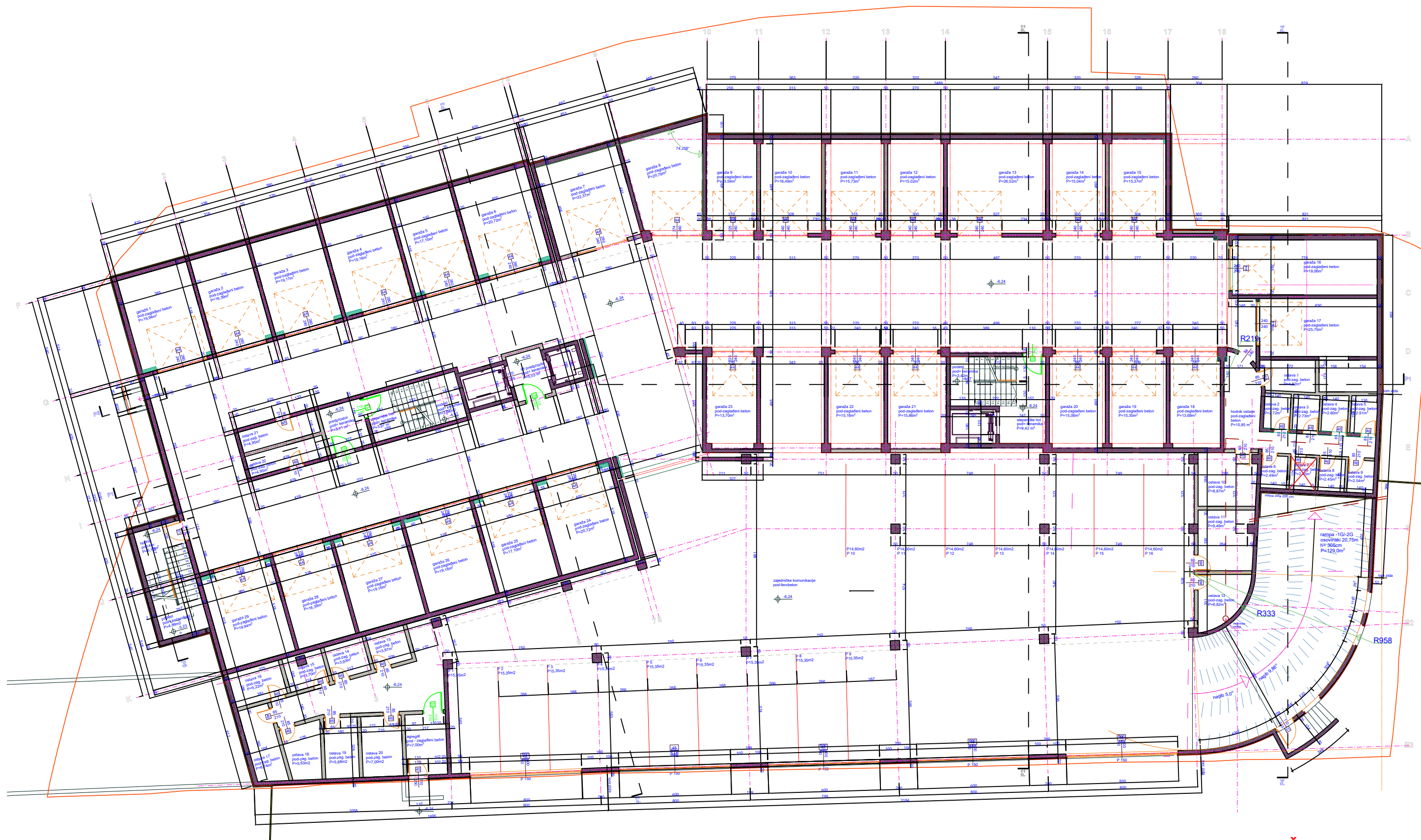
OSNOVA GARAŽA NA KOTI -2
